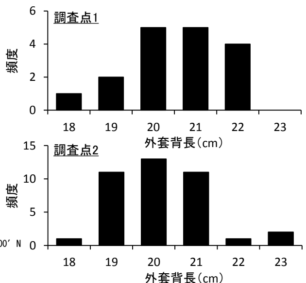
図2 外套背長組成
