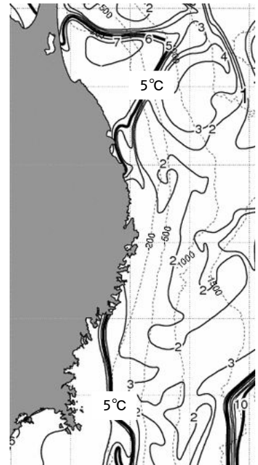
図1 津軽沿岸海域海況日報(3/2) 出典：漁業情報サービスセンター
