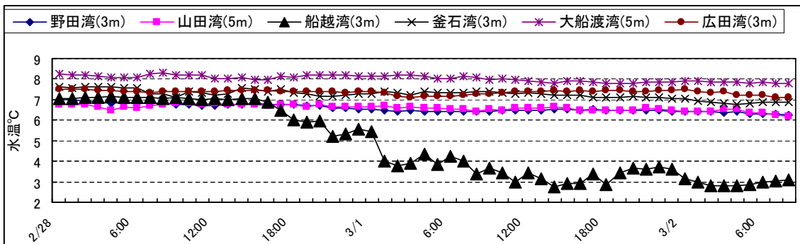
図2 定地水温 各湾の推移（2月28日0:00～3月2日12:00）
