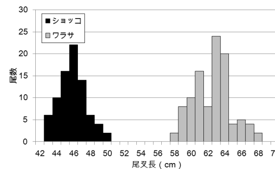
図1 釜石魚市場のブリ体長組成
