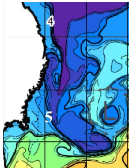
図：3 月 9 日 海況日報 (JAFIC 提供)
