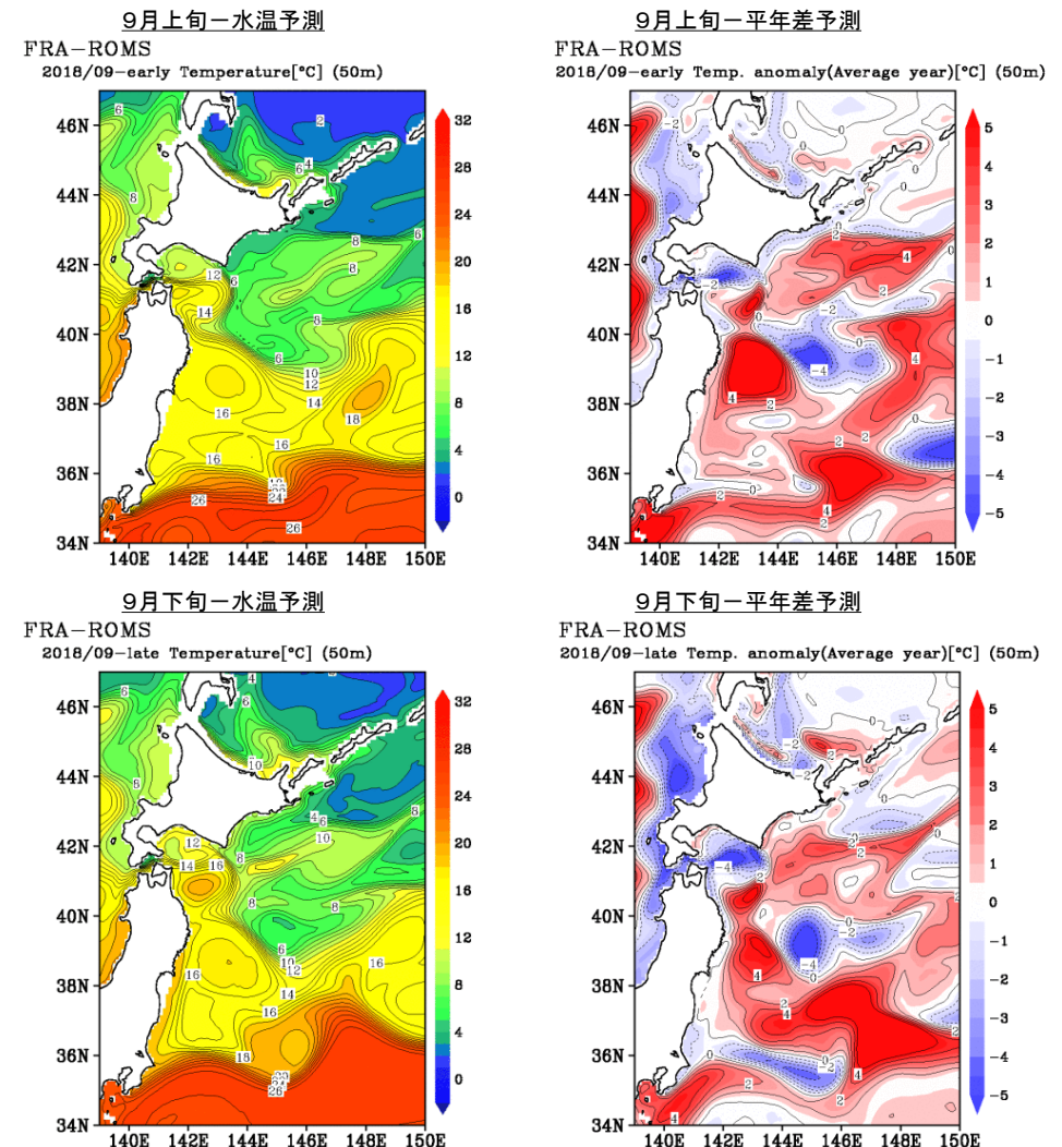
図2 海況予測システムFRA-ROMSによる平成30年9月上旬と下旬の50m深予測水温(左図)および平年差(右図) ※50m深はスルメイカの代表的な分布深度
