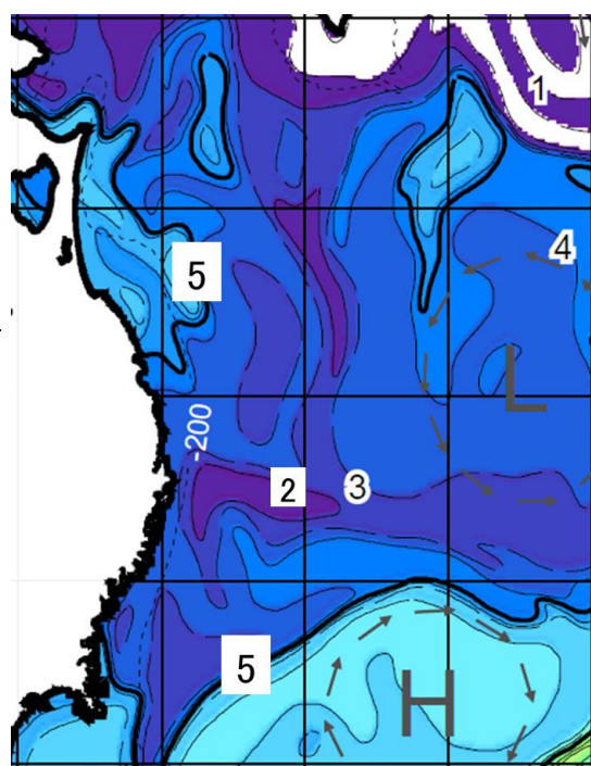
図：海況日報 (JAFIC 提供)
