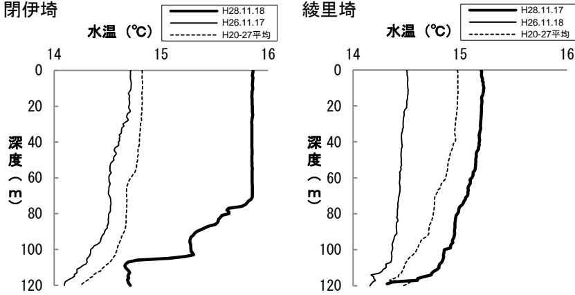
図1 閉伊埼（11月18日）と綾里埼（11月17日）沖の水温観測結果
