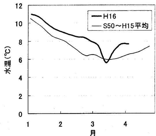
図 船越湾の水深10m層水温
