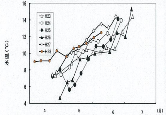
図1 唐丹湾における水深10m層の水温
