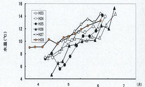
図1 唐丹湾における水深10m層の水溫
