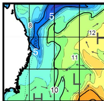
図 2/17 表面水温分布 (JAFIC 発行)
