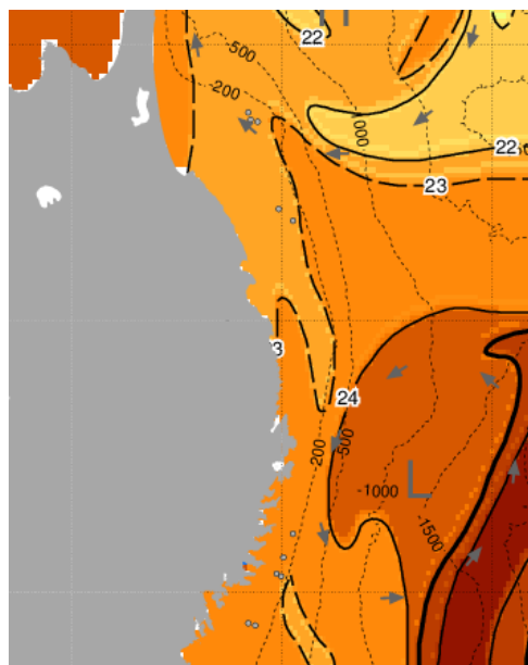
図 8/25表面水温分布 (JAFIC発行)
