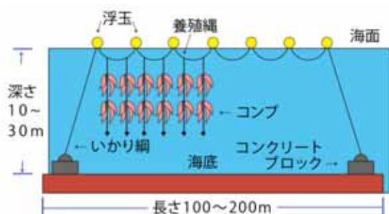
コンプ養殖施設の模式図
