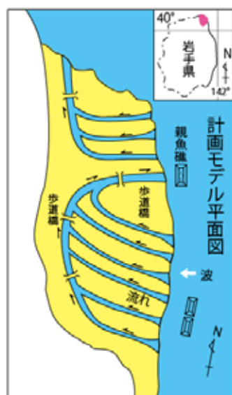
増殖溝方式の増殖場モデル
