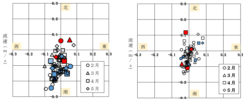
図4：2月から5月の県北部海域（左）、県南部海域（右）の水平流向流速
