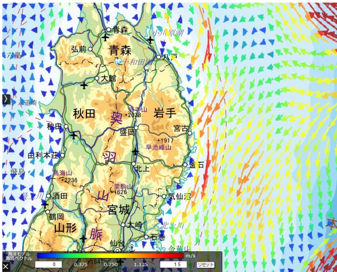
令和6年9月23日12時00分の潮流予想図（表面の解析値） 提供：宇宙航空研究開発機構・海洋研究開発機構（JAXA）
