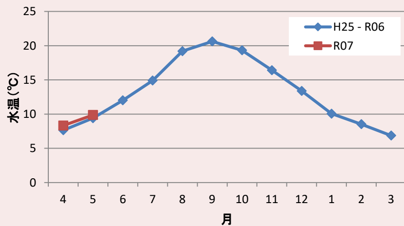
St.3(石浜)_15m層の水溫
