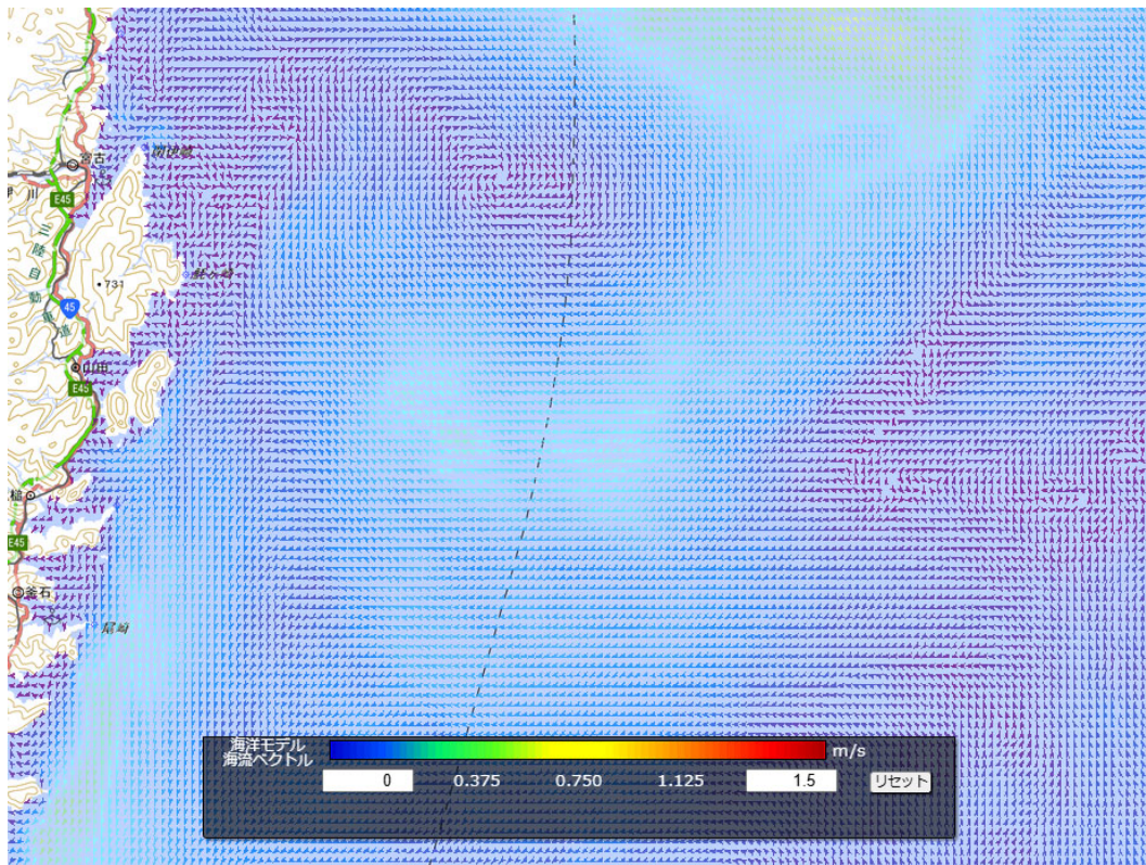
令和7年8月21日24時00分 潮流図（表面の解析値） 提供：宇宙航空研究開発機構・海洋研究開発機構（JAXA）
