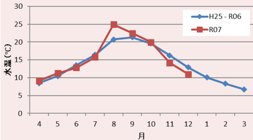
St.4(白浜沖)_5m層の水溫
