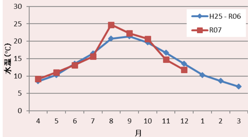
St.1(垂水)_5m層の水温
