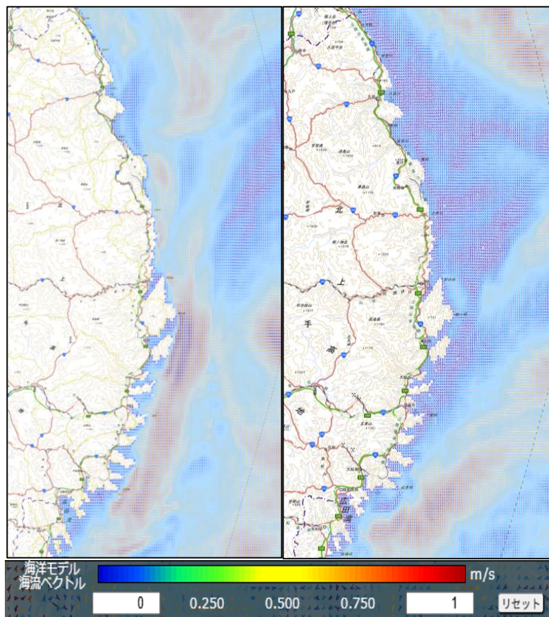
図 表面潮流予想解析図（左：8月21日13時、右：8月23日13時）
